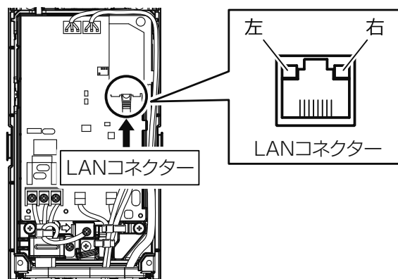
エネルギー計測ユニット
